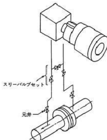
図 5-13 プロセス接続（気体の流量測定）
