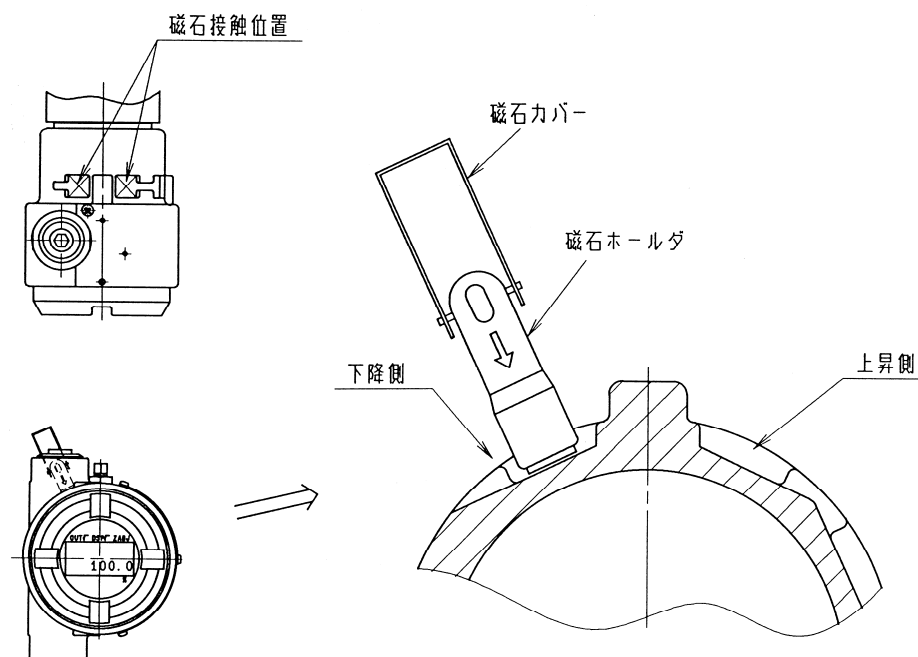
図 8－2 外部調整・設定
