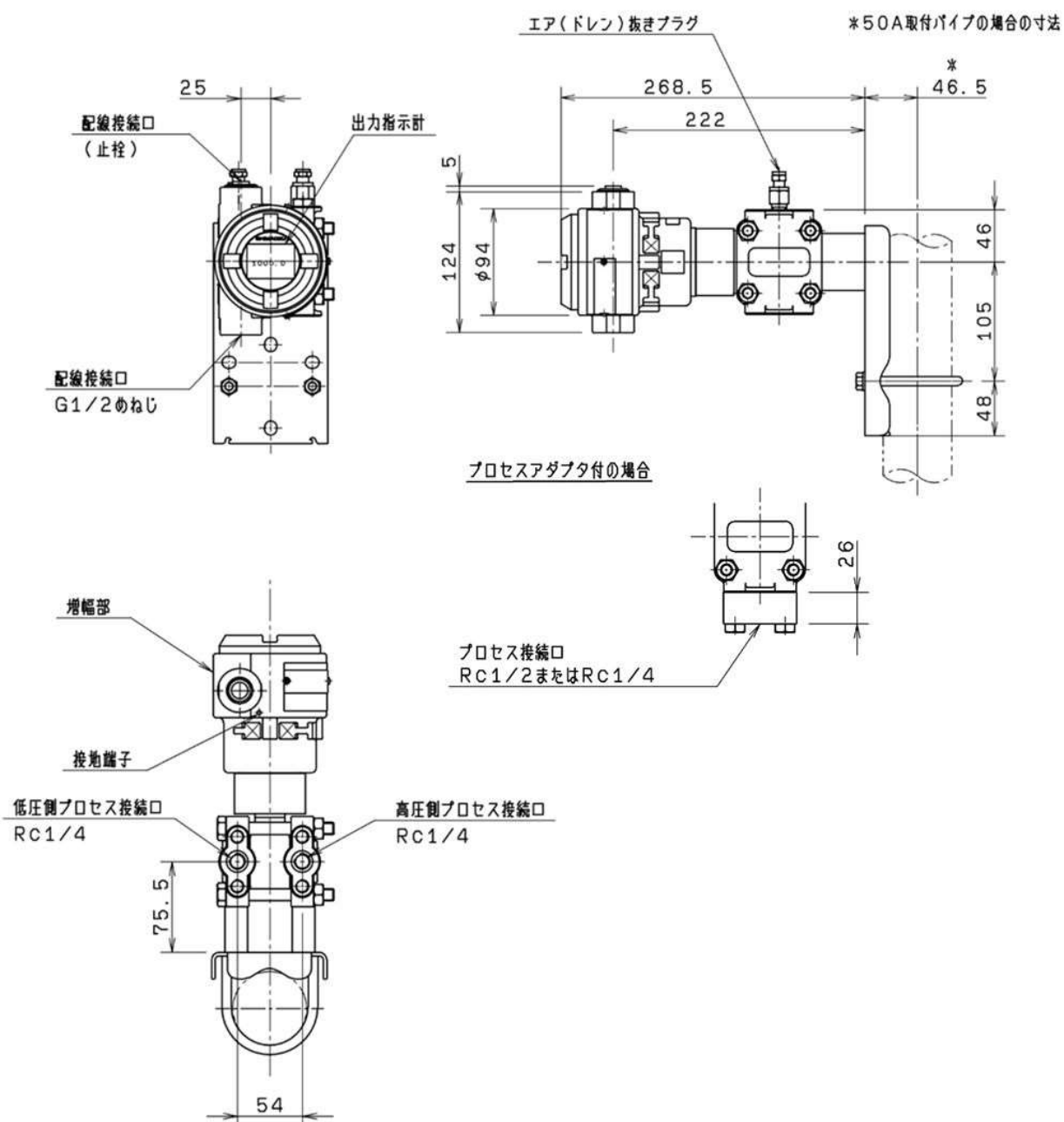
図4-9 T222D, T223D, T224D, T225D 外形図 接液部材質 (ダイアフラム) : SUS316L, ハステロイ C (既設 T122E~T125E(M91), T122D~T125D(M91), T920D, T921D に対するリプレース用)
