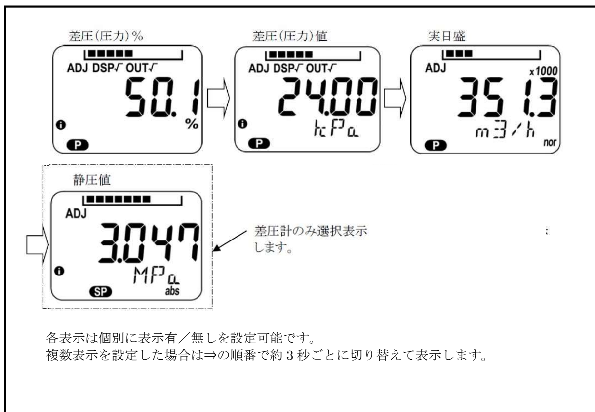
図 7 - 1 3 表示切換
