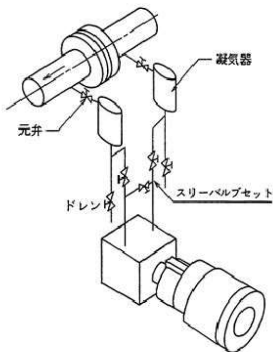
図 5-14 プロセス接続（蒸気の流量測定）
