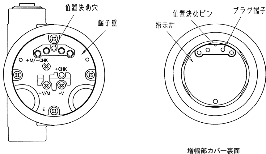
図 5－7 増幅部カバーの取付け，取外し
