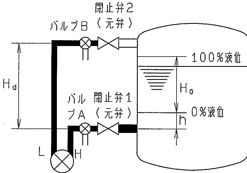
図 6-3 密閉タンクの液位測定配管（ウェット・レグの場合）
