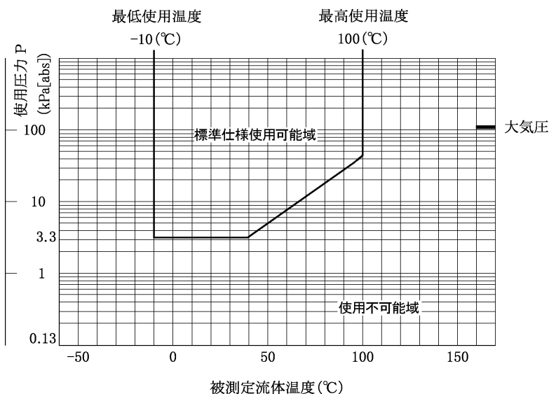
図4-4 使用圧力と接液部温度の関係 (T225D)
