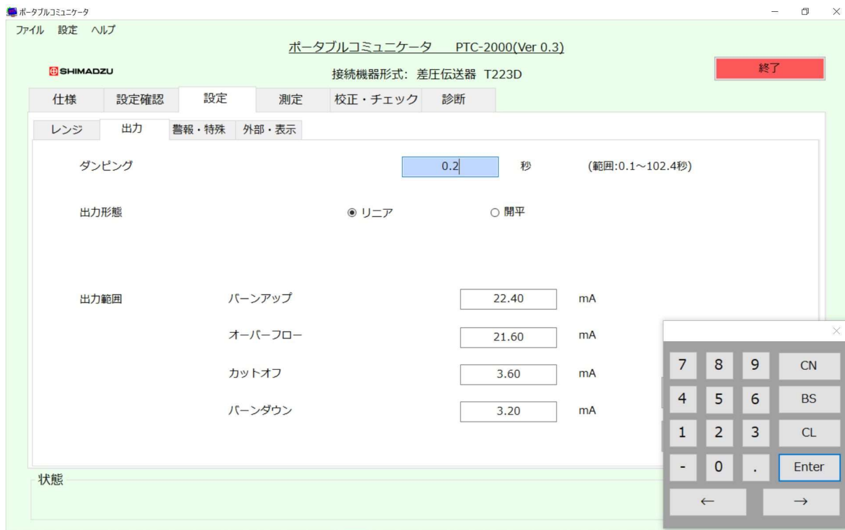
図7-6 数値データ入力
