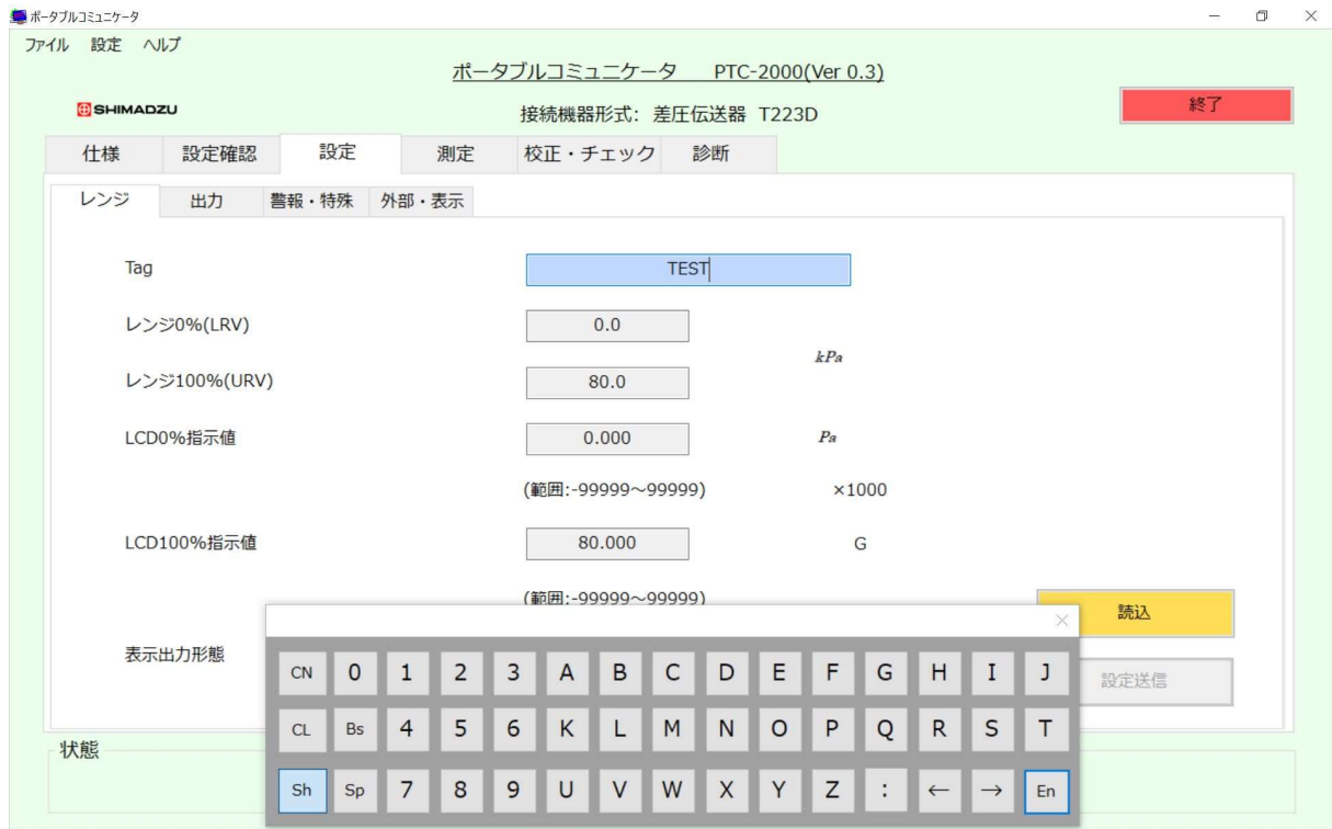
図7-7 文字データ入力
