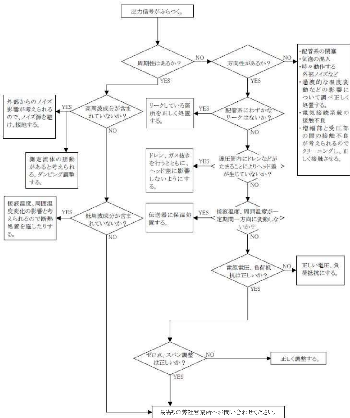
図 9-4 故障箇所判定のフローチャート 4
