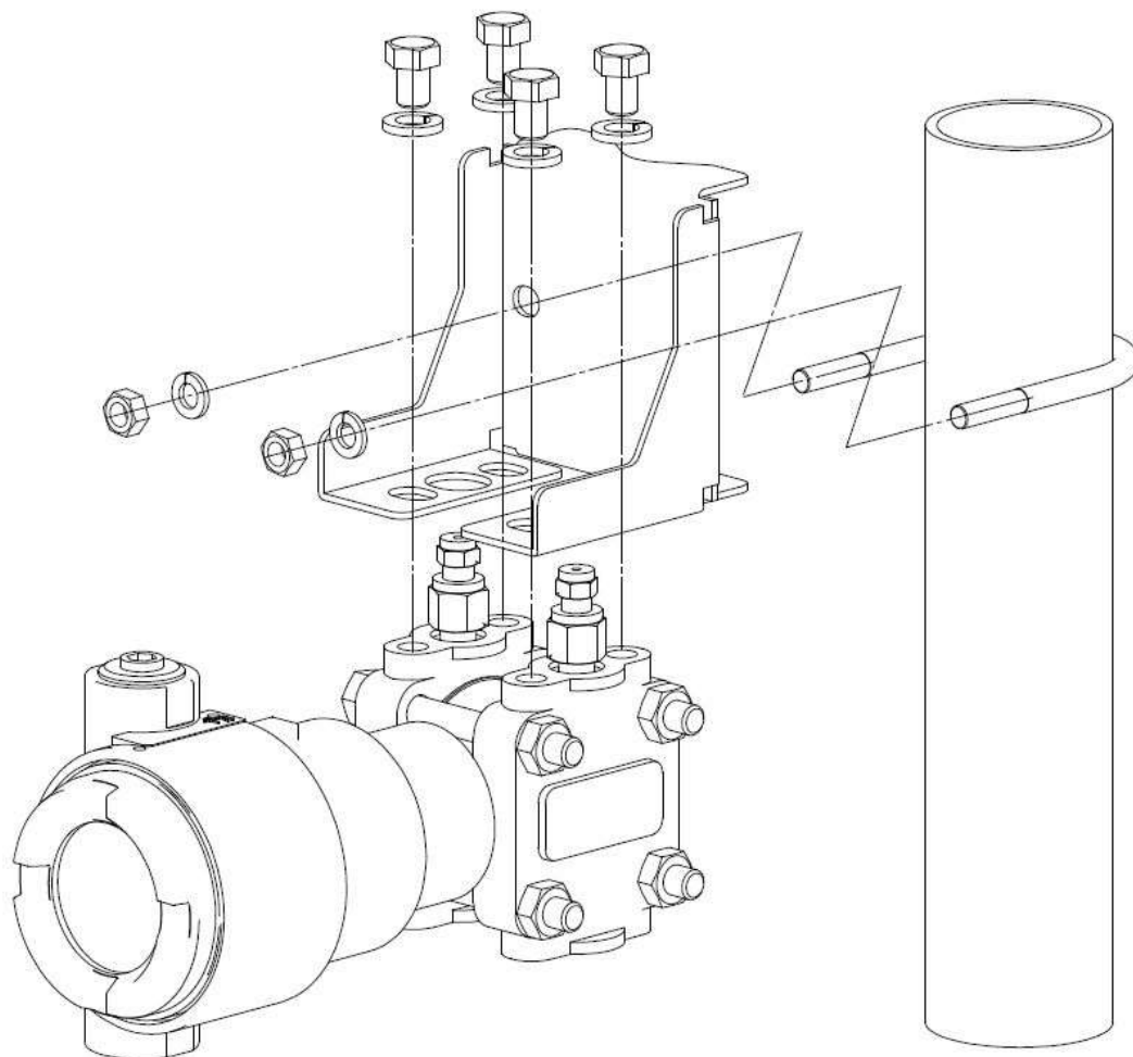
図 5 - 1 伝送器の取付け (T222D～T225D)
