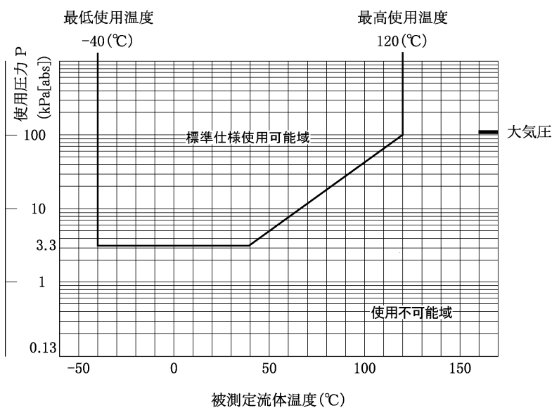
図4-3 使用圧力と接液部温度の関係 (T222D, T223D, T224D)
