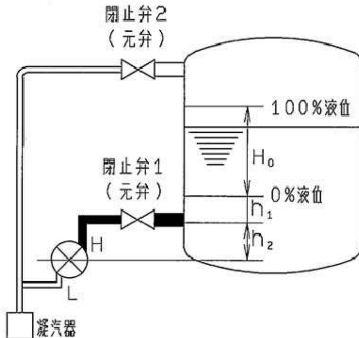
図6-2 密閉タンクの液位測定配管（ドライ・レグの場合）
