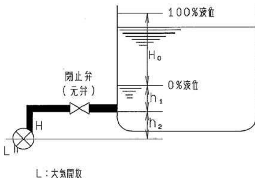
図6－1 開放タンクの液位測定配管
