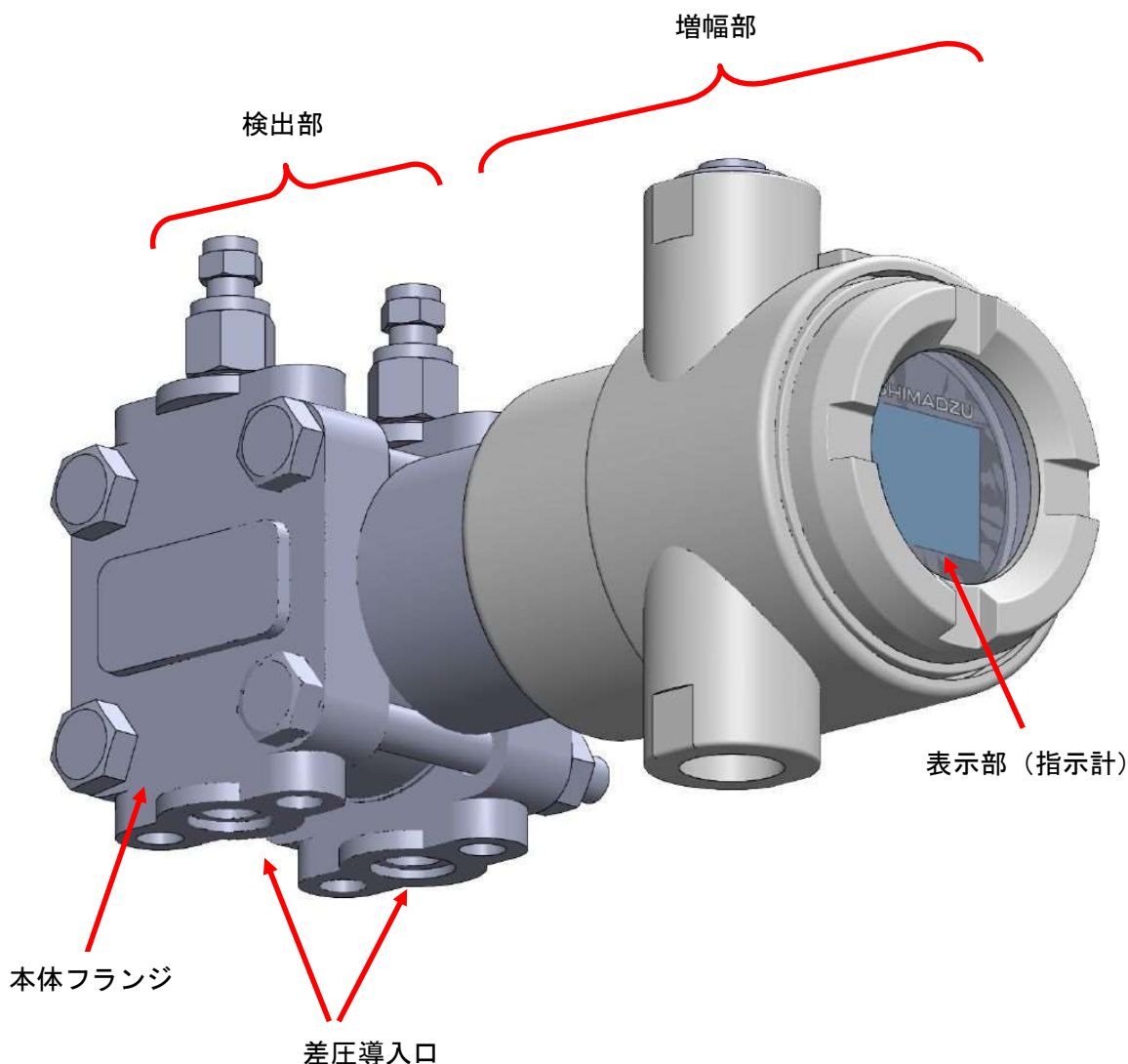
図 2 - 1 伝送器の各部名称
