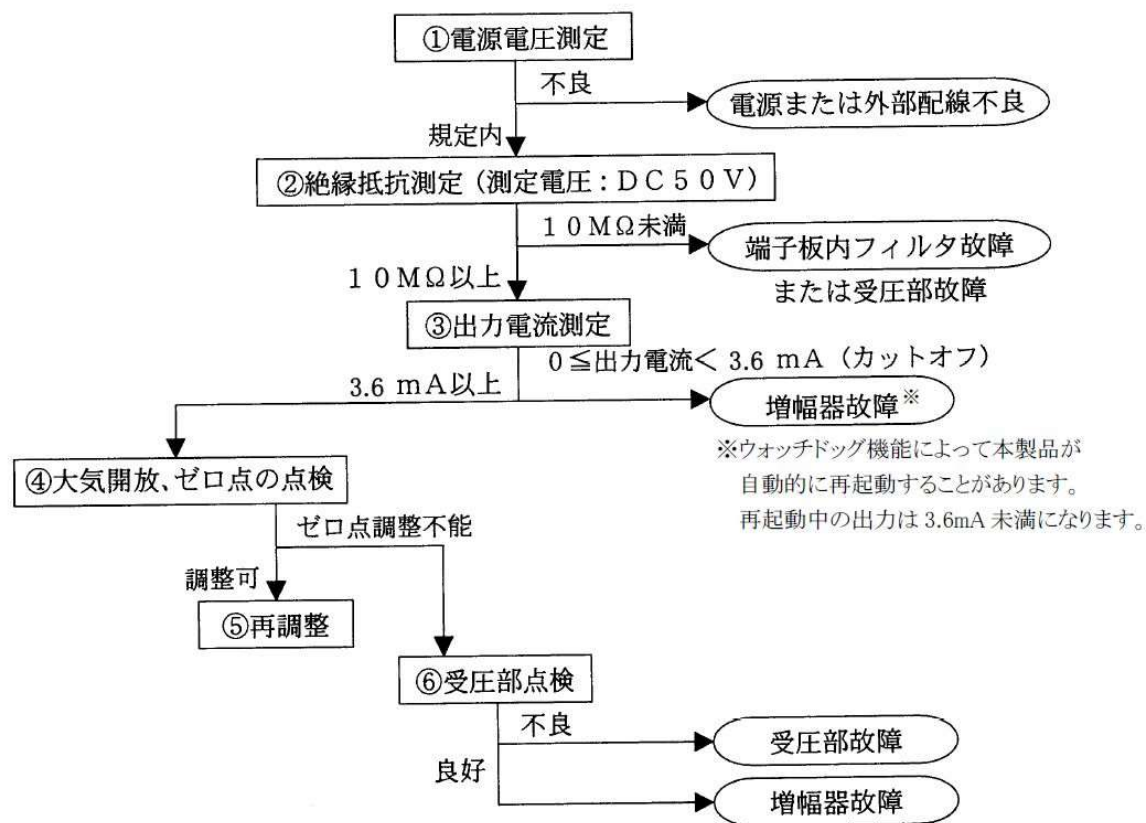
図9-1 故障箇所判定のフローチャート1
