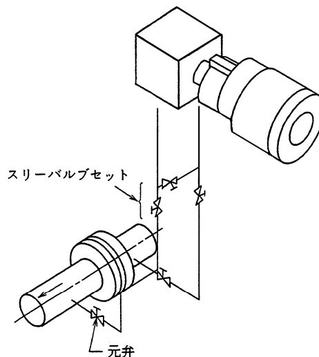
図 5-12 プロセス接続（液体の流量測定） 配管より上に取り付の場合
