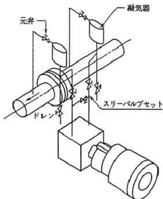
図 5-15 プロセス接続（蒸気の流量測定）
