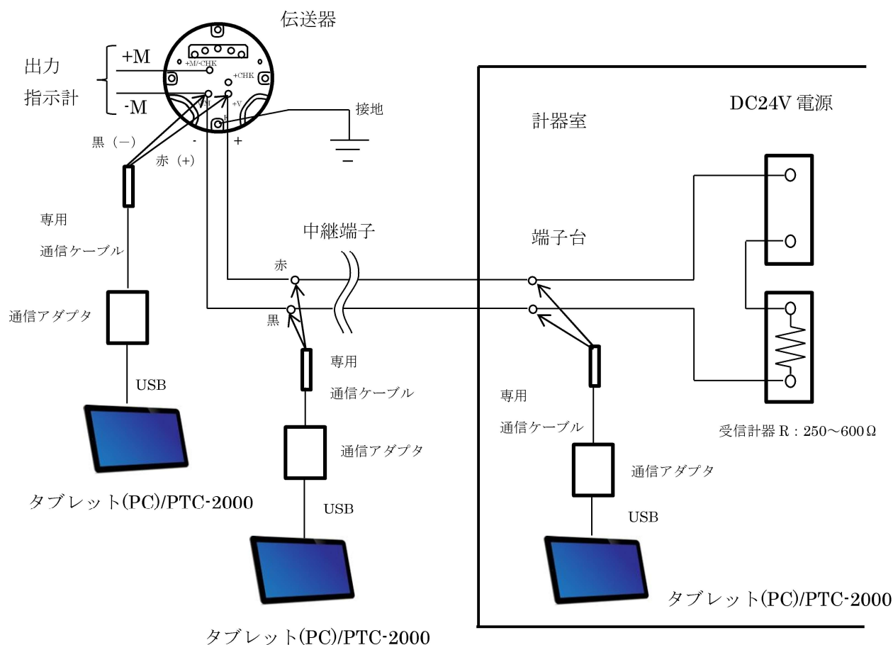
図 7－1 接続例
