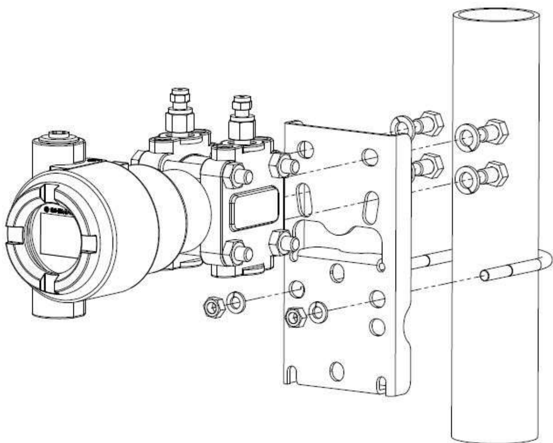
図 5 - 2 伝送器の取付け (FT) (T222D~T225D)
