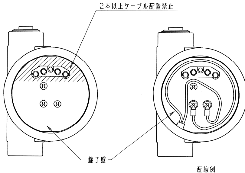
図 5－6 配線接続図
