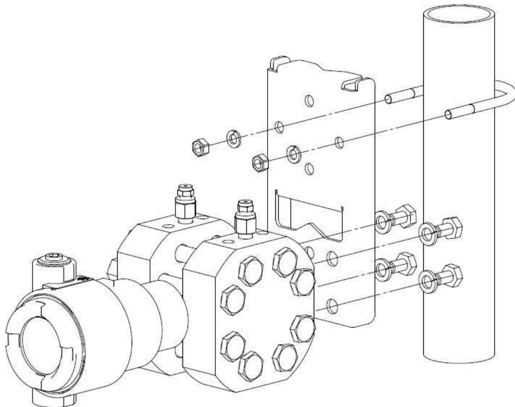
図 5 - 3 伝送器の取付け (T228D, T229D)
