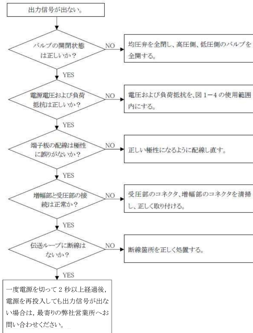
図 9-2 故障箇所判定のフローチャート 2
