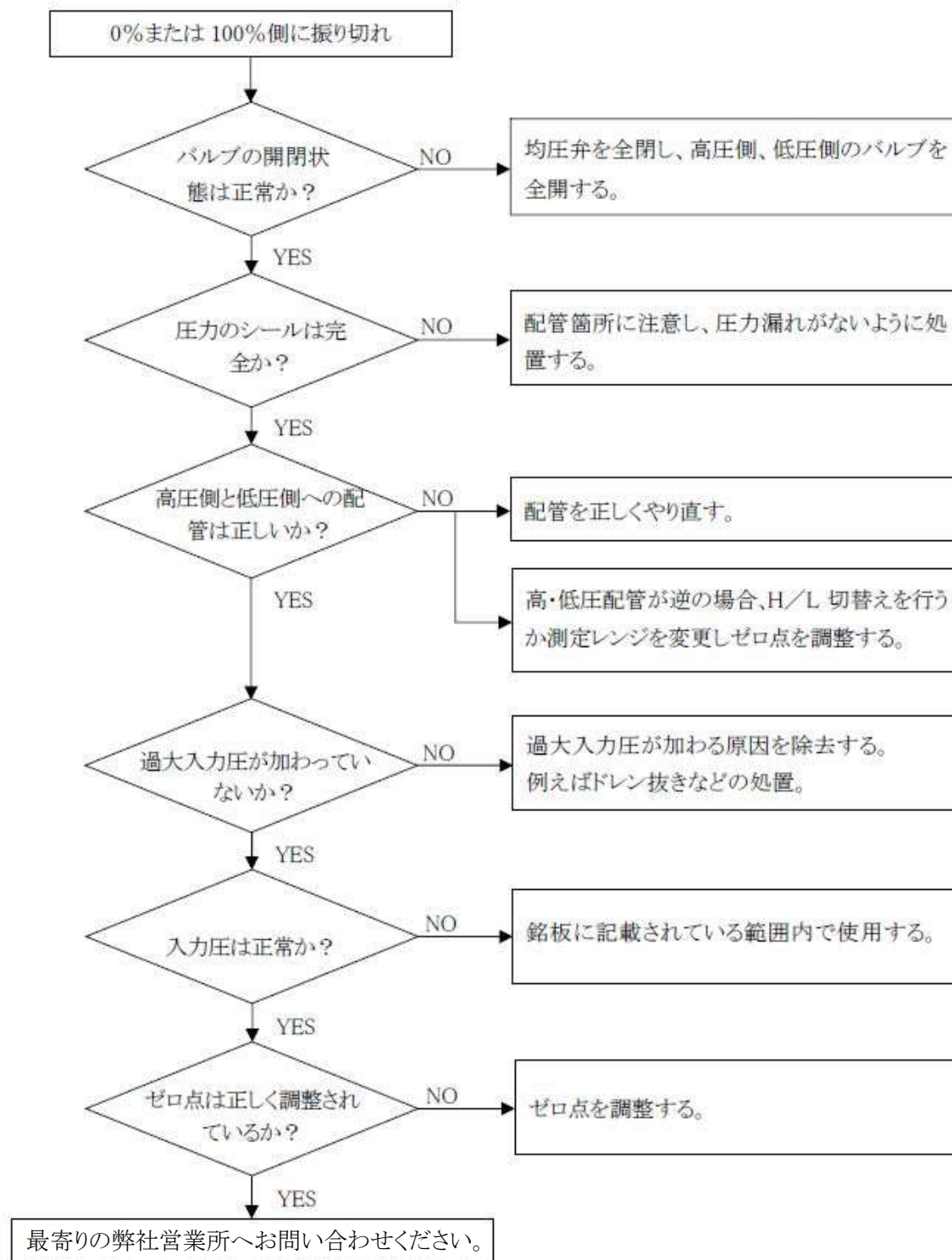
図 9-3 故障箇所判定のフローチャート 3
