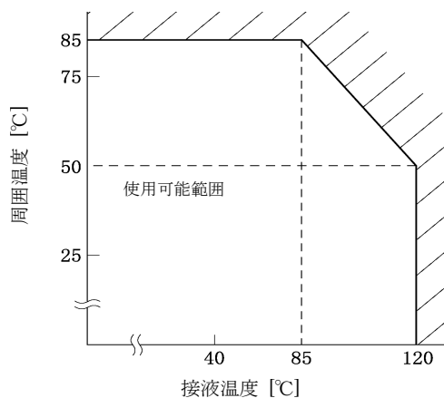
図 4 - 2 使用周囲温度と接液部温度の関係
