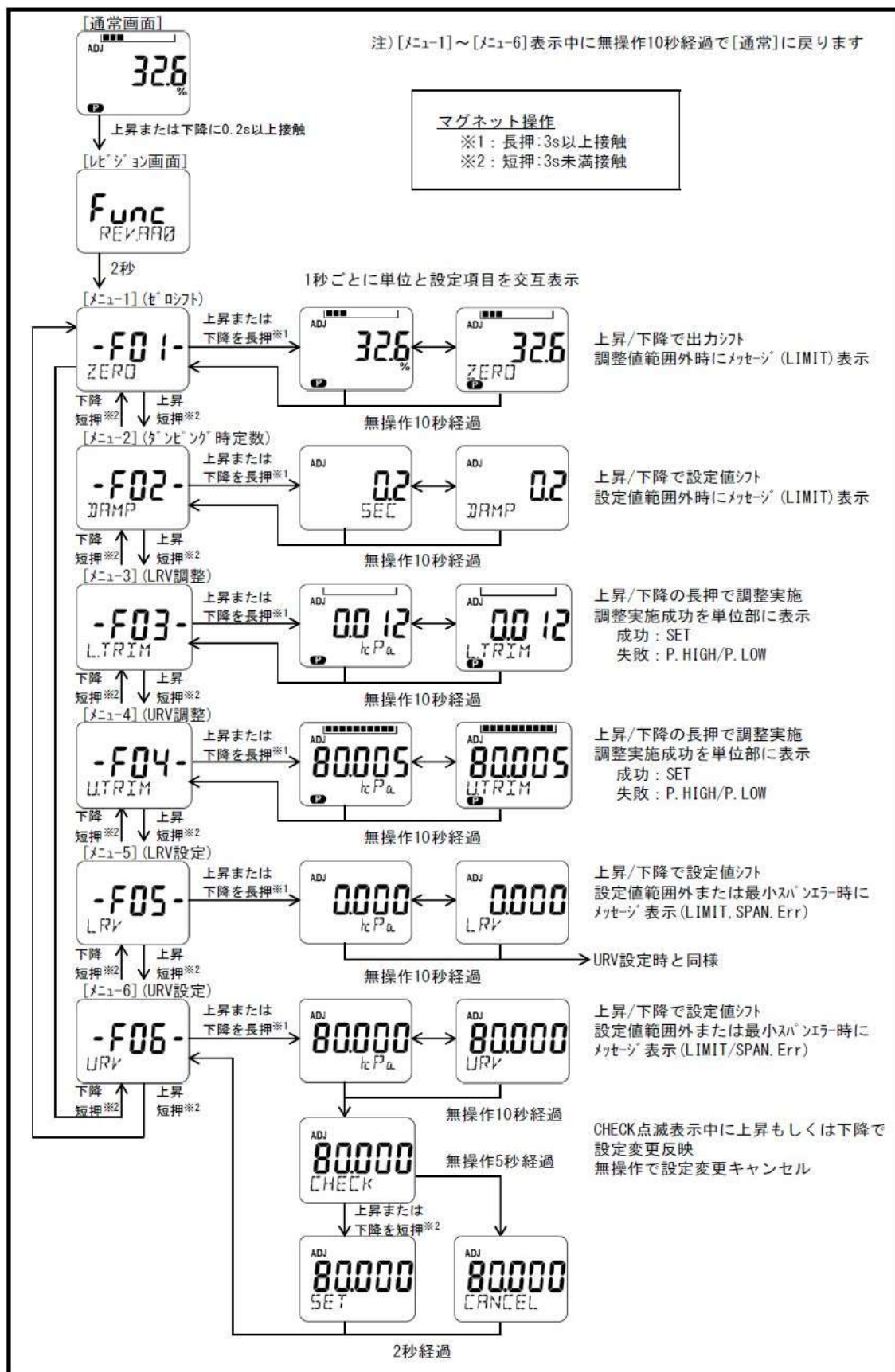
図 8 - 3 画面展開図
