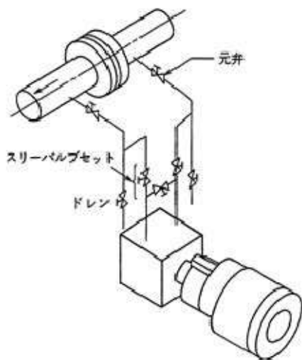
図 5-11 プロセス接続（液体の流量測定） 配管より下に取り付の場合
