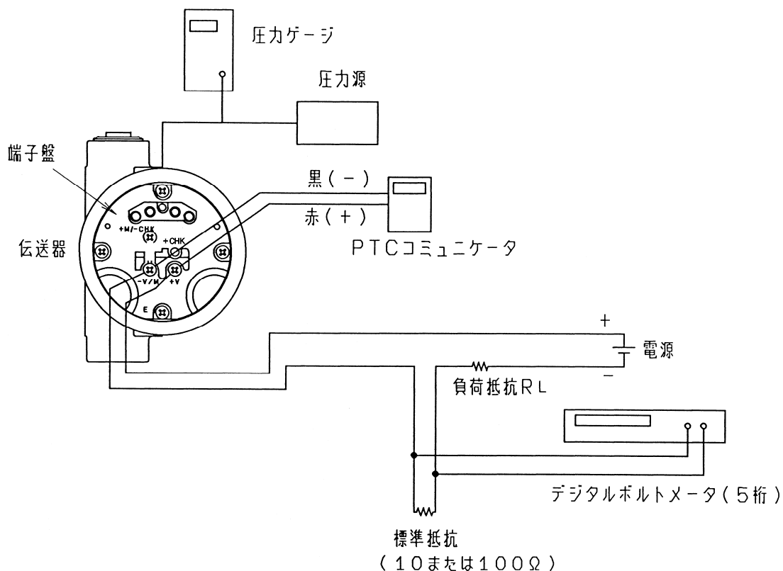
図8-1 接続図
