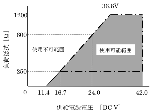
図 4－1 伝送器電源電圧／負荷抵抗特性
