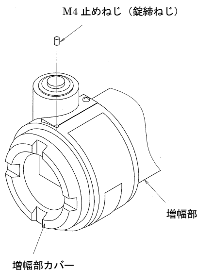
図 5 - 5 錠締
