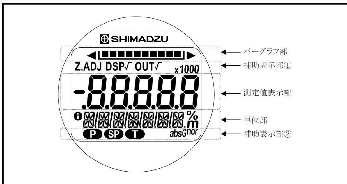
図 7-1 2 指示計の画面構成
